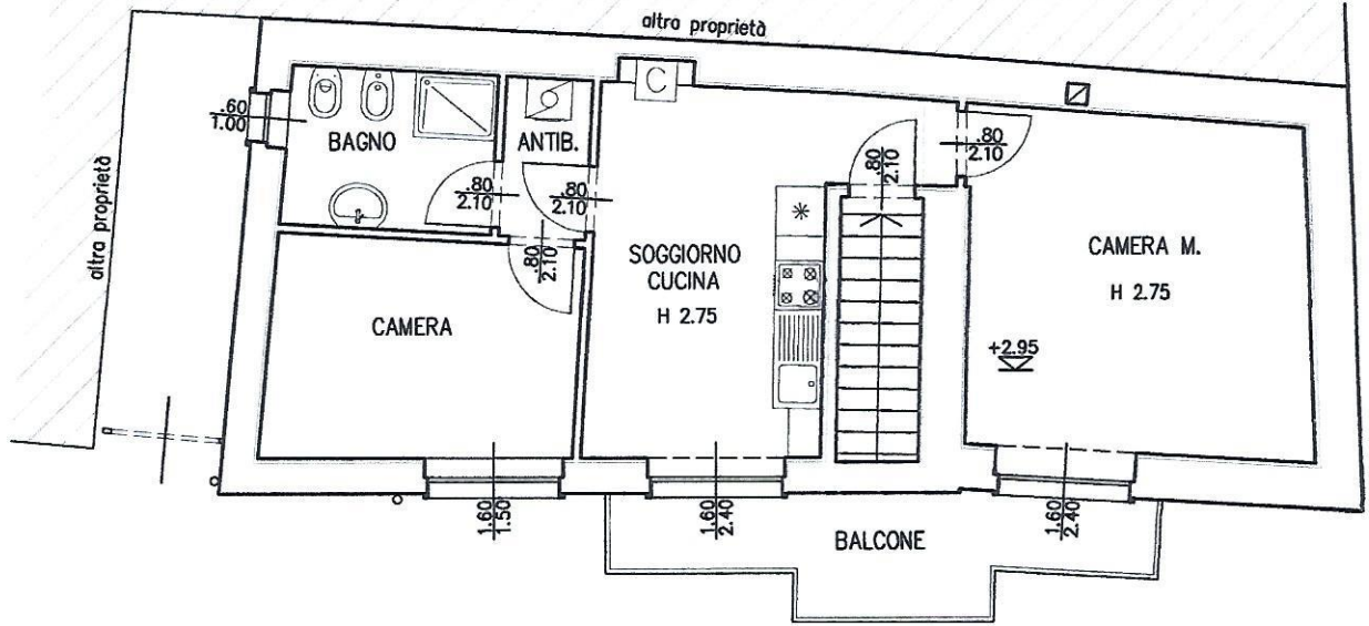
PIANO PRIMO RAPP. 1:100
